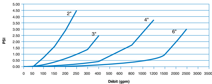
Perte de charge : 2" à 6"
