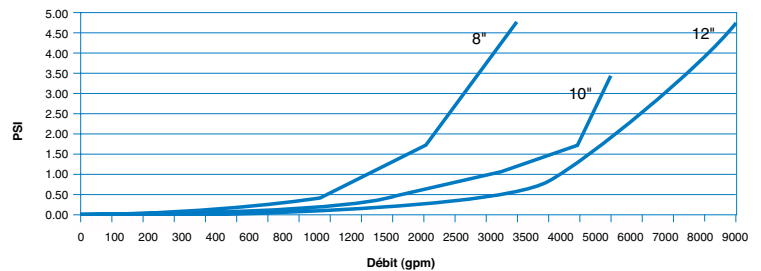
Perte de charge : 8" à 12"
